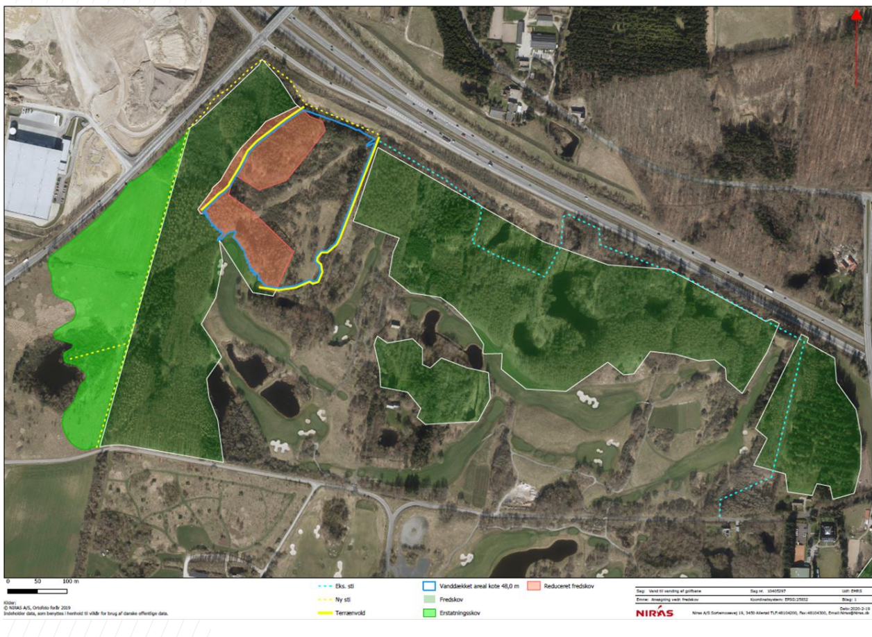
Figur 5.1: Placering af nyt reservoir
